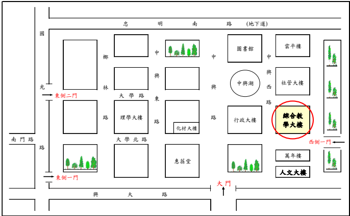
【試場平面圖】
