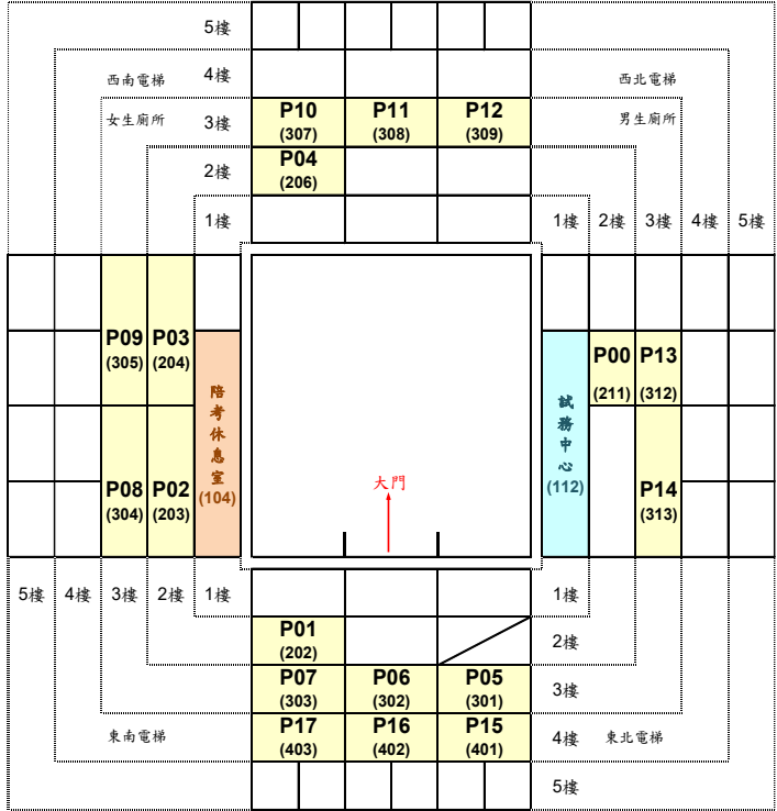
【試場平面圖】
